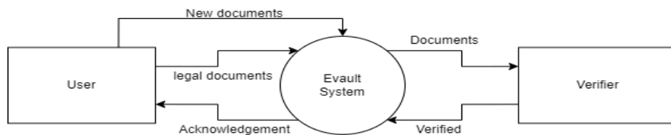
Fig 4.2.1 Level 0 DFD
